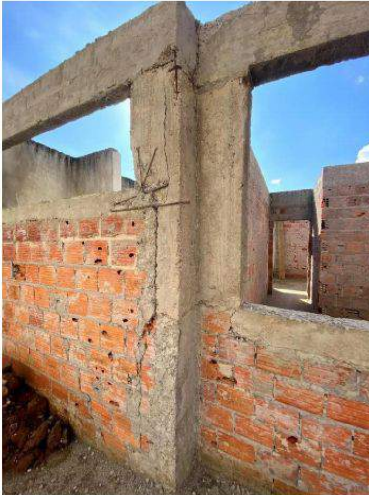
Descolamento da alvenaria junto a estrutura e ferragem exposta
